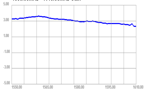
1550.00MHz - 1610.00MHz Gain
