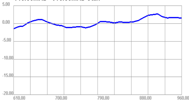
610.00MHz - 960.00MHz Gain
