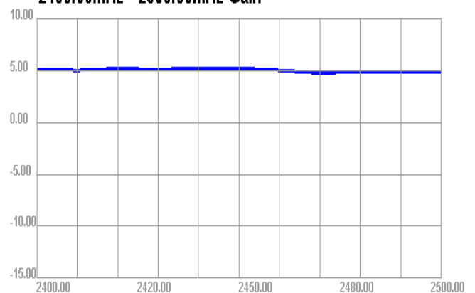
2400.00MHz - 2500.00MHz Gain
